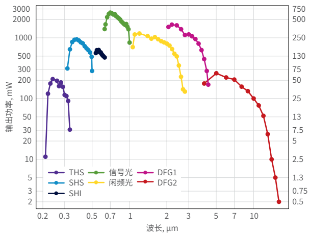
ORPHEUS-HE-5mJ 的典型调谐曲线 泵浦: 20 W, 5 mJ, 4 kHz
